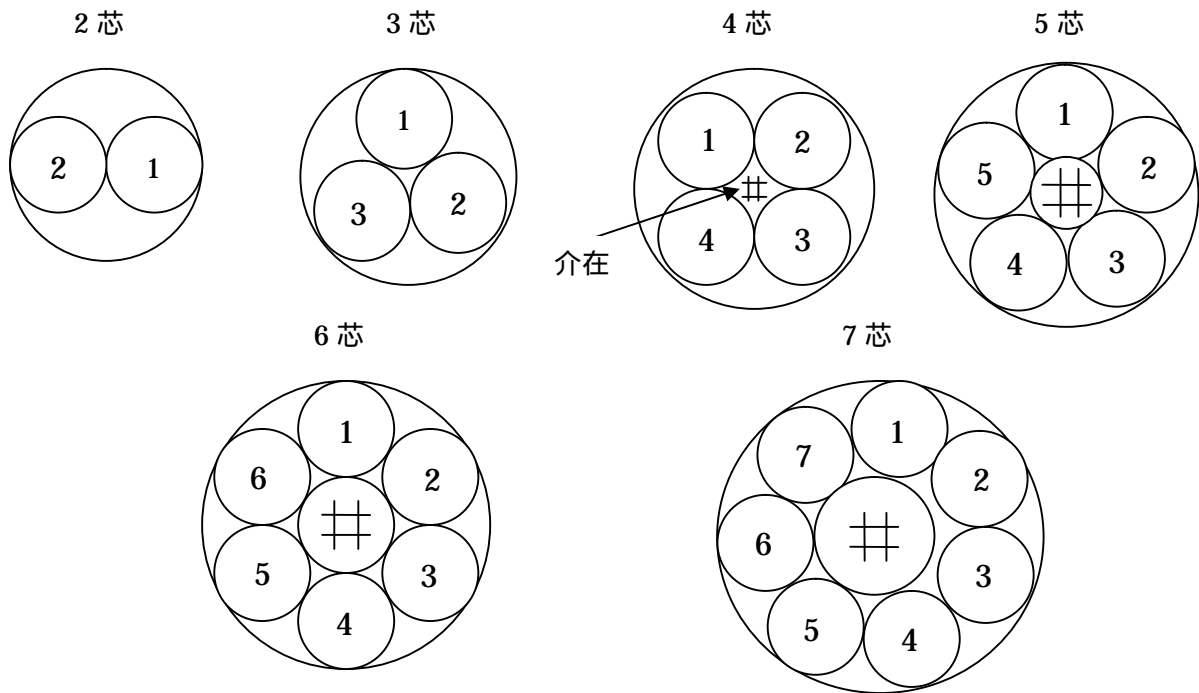
図 1 配列図
